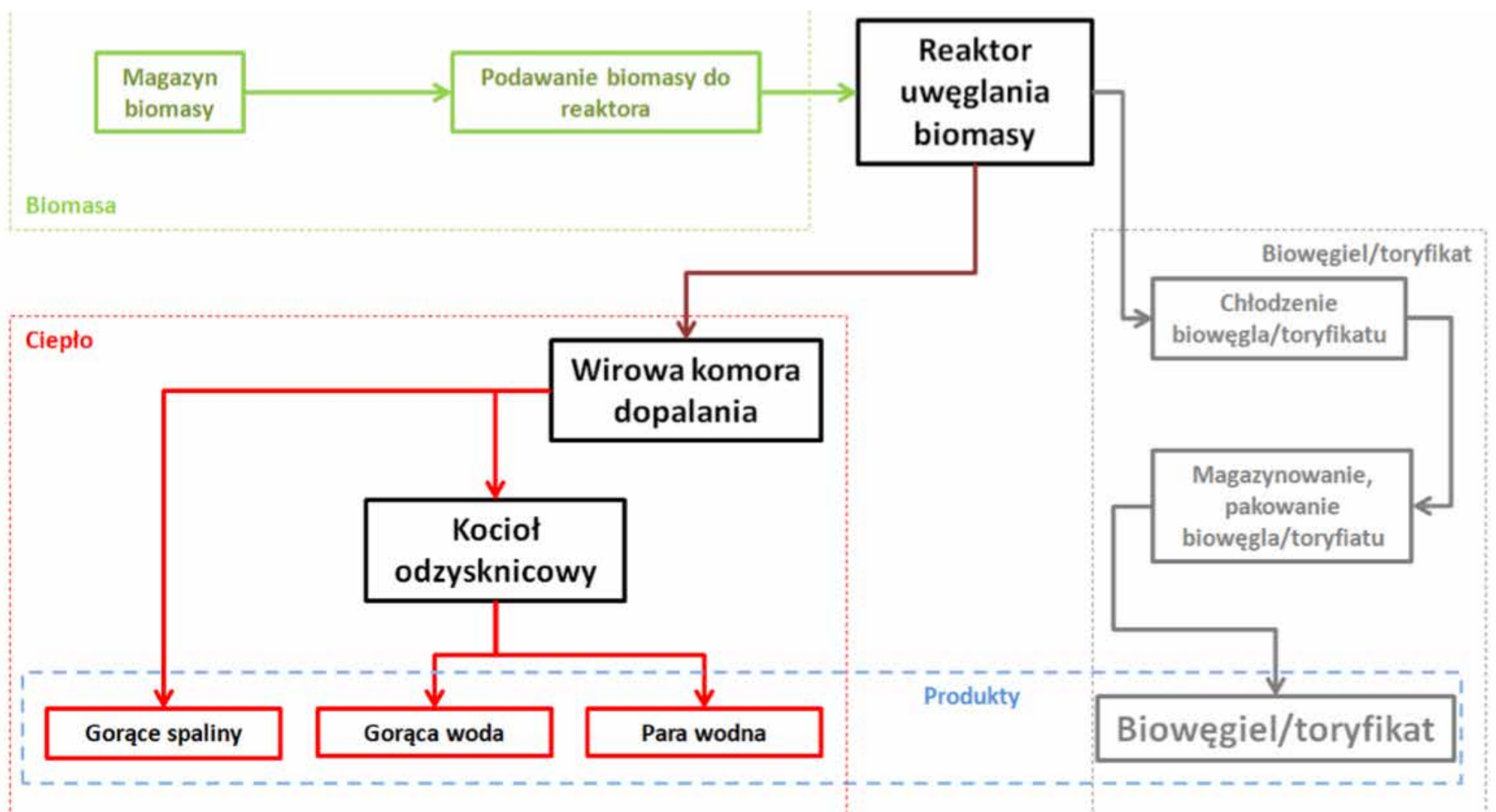
Rys. Schemat technologiczny termicznego przetwarzania biomasy (opracowanie własne)
