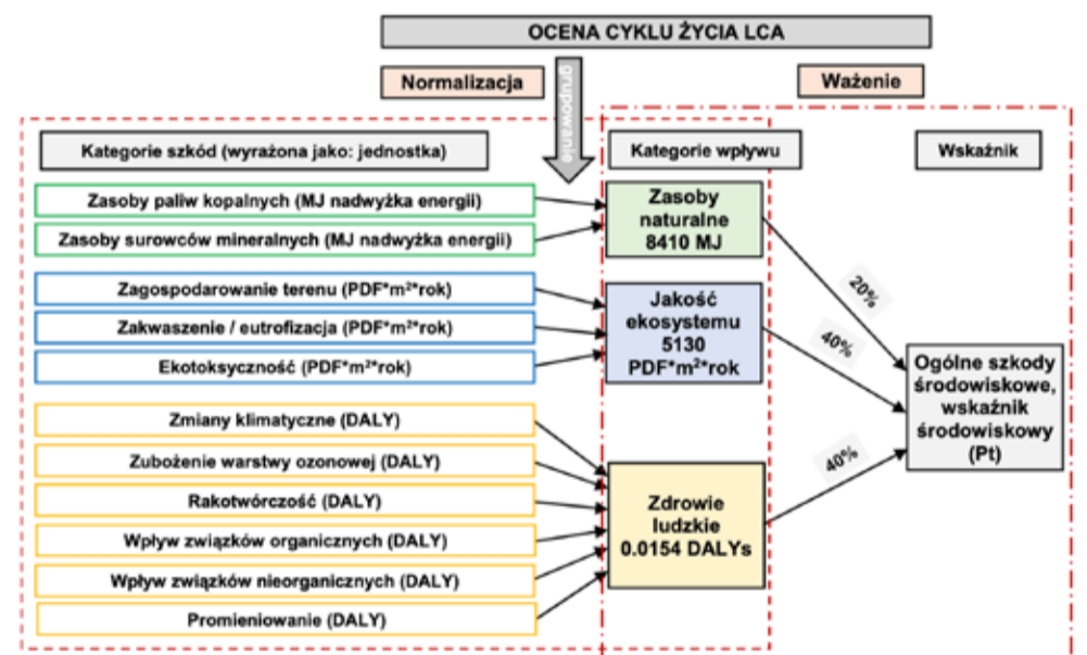
Rys. 1. Kategorie szkód i odpowiadające im kategorie wpływu w ocenie cyklu życia LCA (Opracowanie własne)
