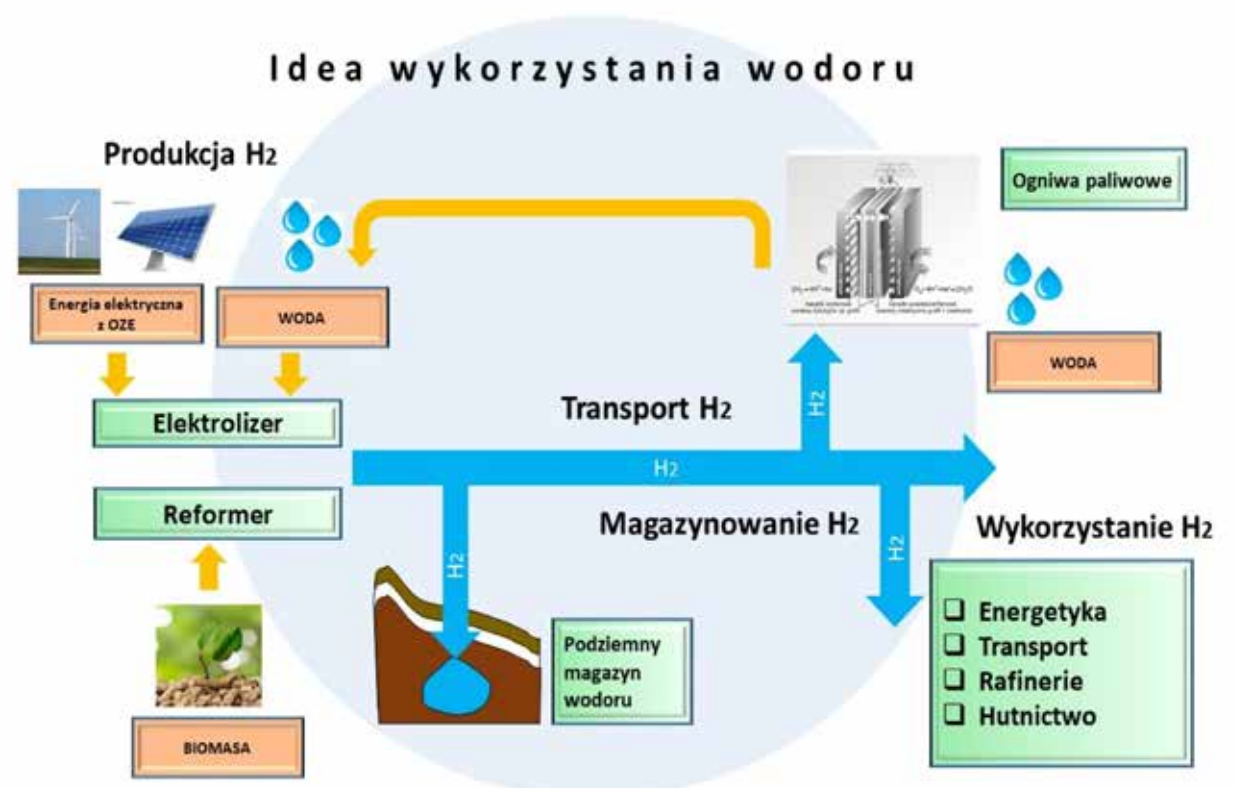
Rys. 1. Przykład systemu hybrydowego ogniwo paliwowe + ogniwo fotowoltaiczne + elektrolizer [2]
