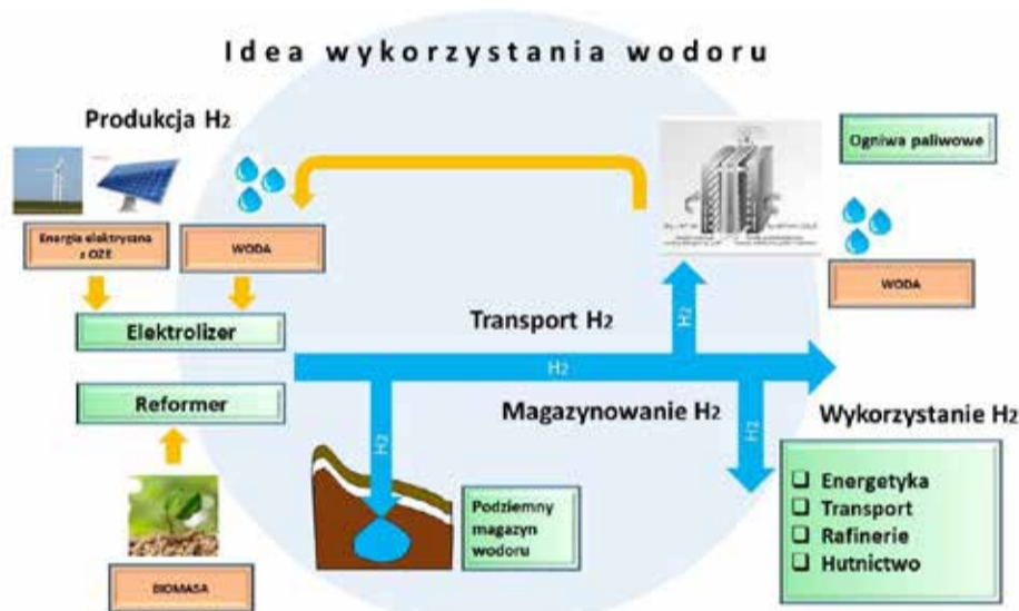
Rys. 1. Przykład systemu hybrydowego ogniwo paliwowe + ogniwo fotowoltaiczne + elektrolizer [2]
